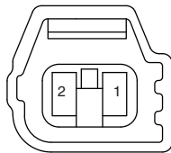
DPF Temp T1 Sensor (U10)
