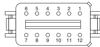
WCU J1 ( U19 ) (Black)
